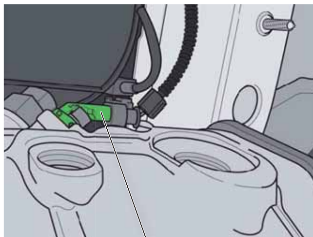
датчик нейтрального положения КП G701
